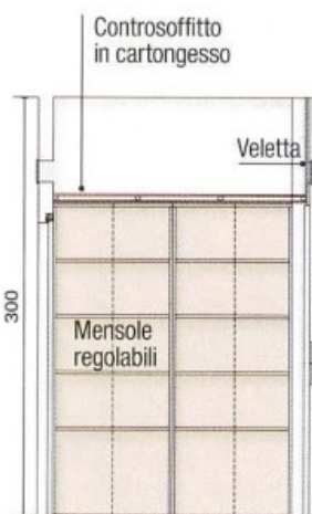
PROSPETTO DELL'ARMADIO APERTO
